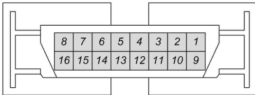
ECU OBD-II 단자정보
