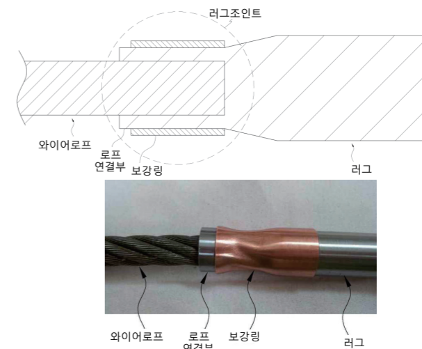
[ 본 기술에 따라 제조된 러그 조인트의 도면 ]
