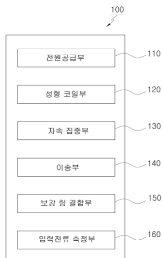
[ 본 기술에 따른 러그 조인트 성형장치의 블록도 ]
