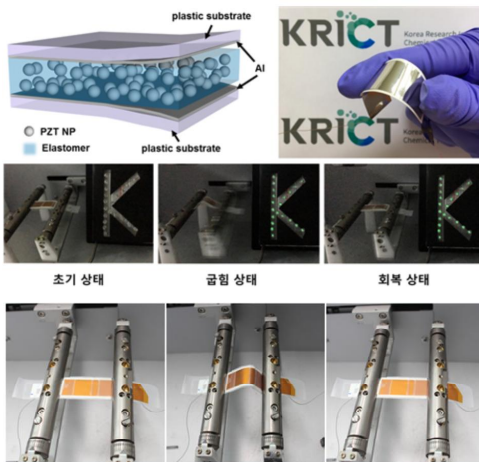
[KRICT 유연 압전소재] 굽히는 힘에 의해 균일하게 분포된 압전 입자구조가 구부러졌다 펴지는 과정에서 전기에너지 발생
