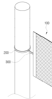
< 실외용 미세먼지 제거장치 도식화 >
