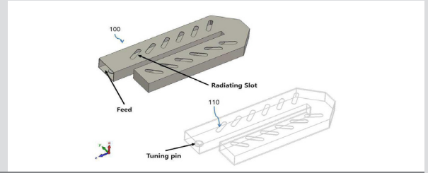
마이크로웨이브 가열용 진행파형 직각 도파관 도면 ▲
