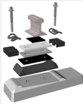
KR형 레일체결장치
