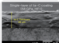
고경도 DLC 공정 기술
