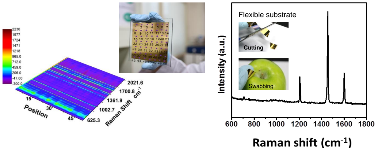
SERS 기판의 대면적 균일성을 보여주는 데이터 (좌) 및 사과 표면의 농약검출 결과
