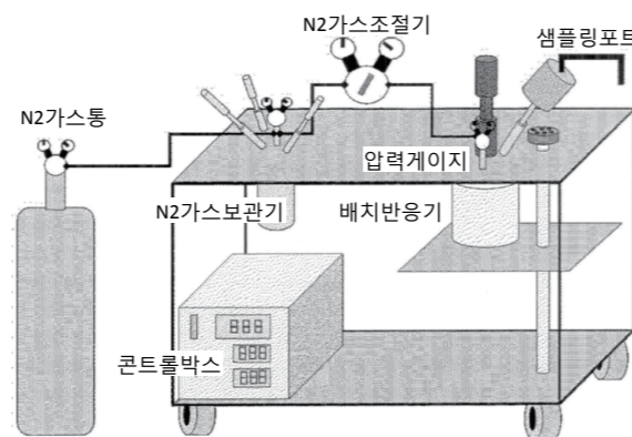
[ 당화장치의 개략도 ]
