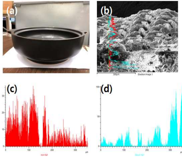
[(a) 제작된 샘플, (b) 결합부 SEM 분석 이미지, (c) EDS 분석 결과 (Fe), (d) EDS 분석결과 (Si) ]
