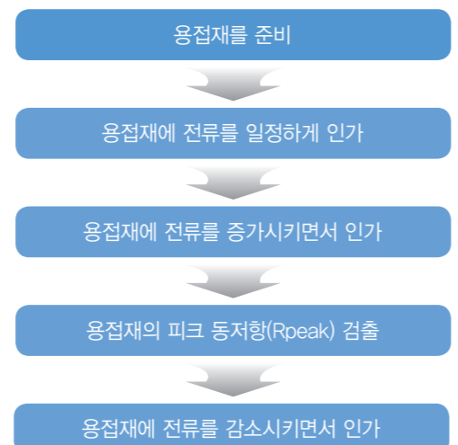
【 본 기술에 따른 용접제어 방법 】
