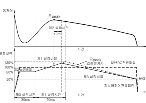
【 동저항 검출 과정에 따른 전류인가 수준을 예시한 그림 】
