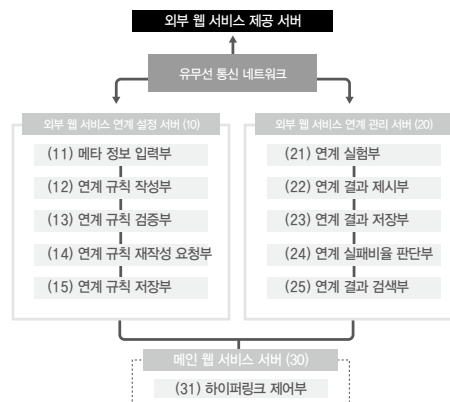
웹 서비스 연계 관리 시스템의 구성 도면
