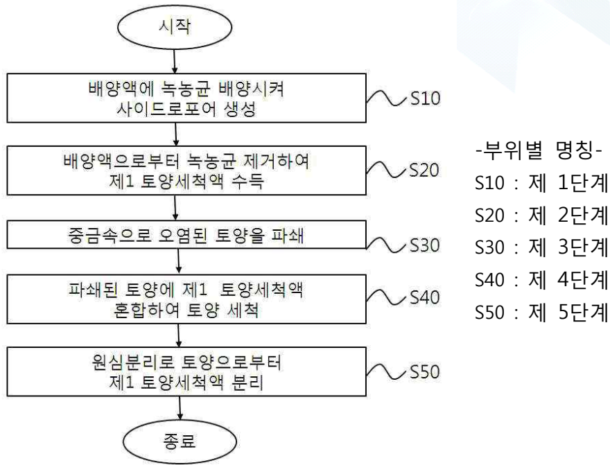
<그림> 중금속으로 오염된 토양의 세척방법의 흐름도
