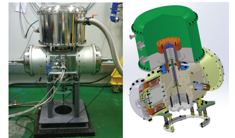
[대용량 스텐링 극저온 냉동기]
