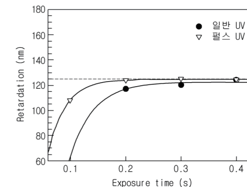
[ 노광시간에 따른 광배향층의 위상차 변화 비교 ]
