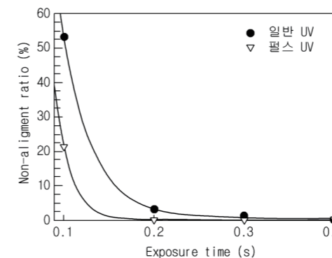
[ 노광시간에 따른 광배향층의 미배향 분포도 비교 ]
